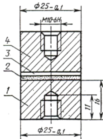
1 — образец; 2 — покрытие; 3 — клеевая прослойка; 4 — контробразец
